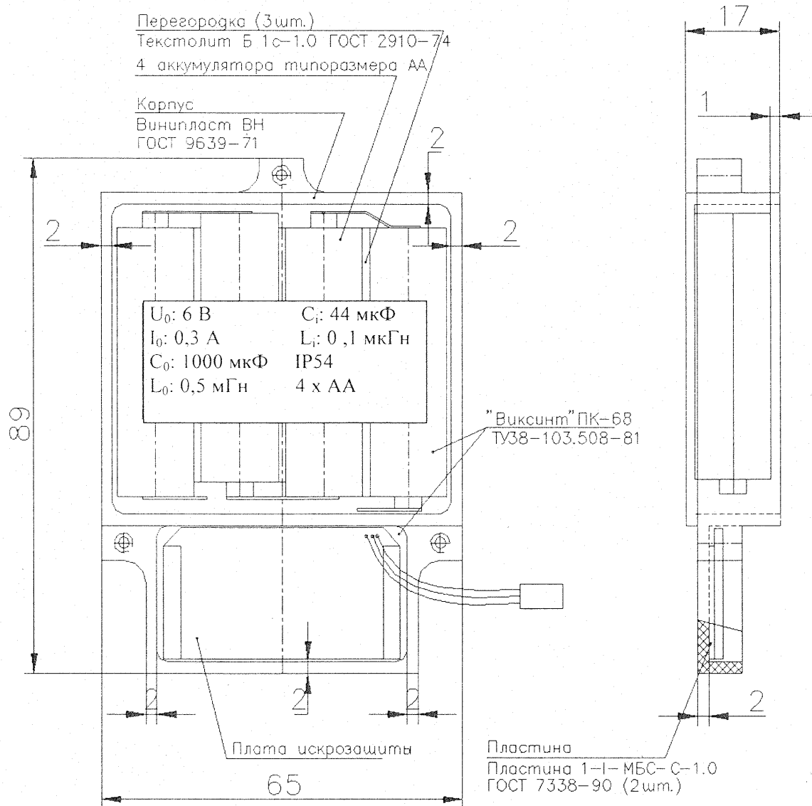
Рисунок 4.3 – Чертеж средств взрывозащиты блока питания
