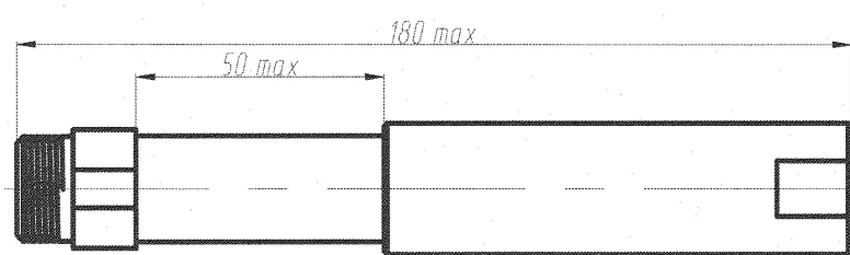
Рисунок 1 - Сгон БС-25-01, БС-25-02
