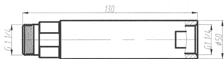
Рисунок 1 - Сгон БС-25-01, БС-25-02
