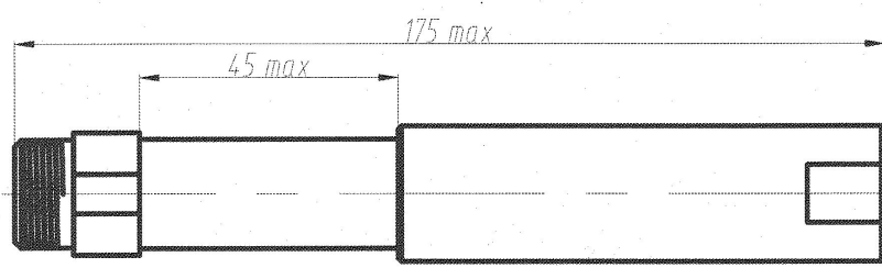
Рисунок 2 - Сгон БС-32-01, БС-32-02
